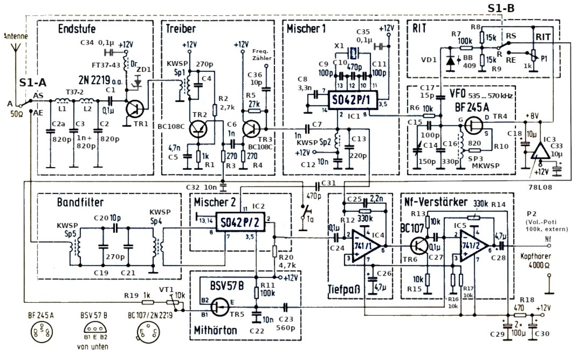
Bild 2. Vollständiges Schaltbild des Transceivers für das 80-m-CW-Band
