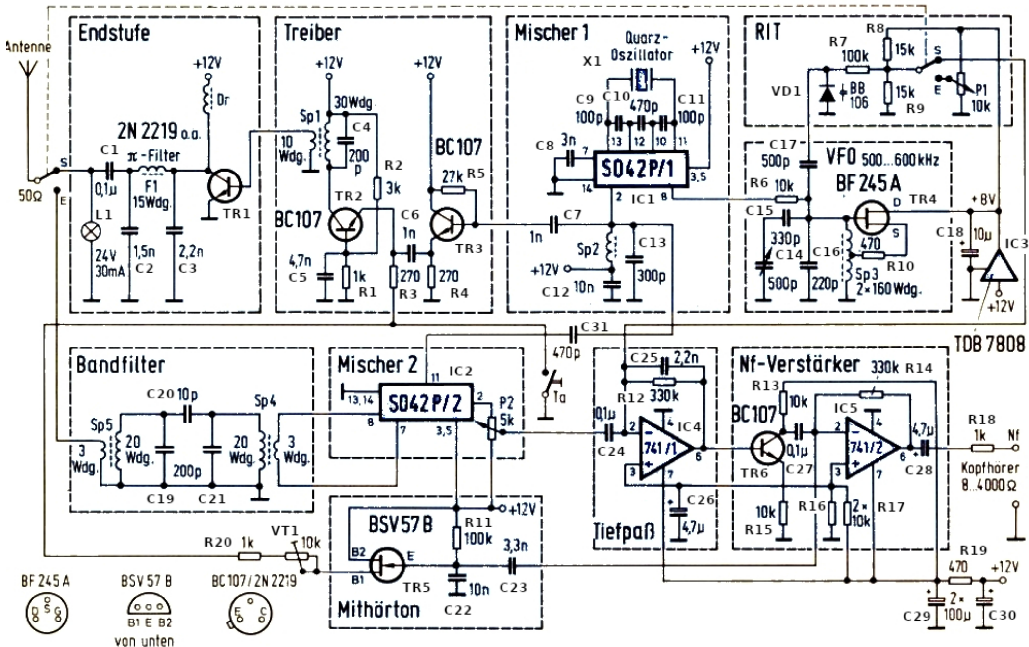
Bild 2. Vollständiges Schaltbild des Transceivers für das 80-m-CW-Band
